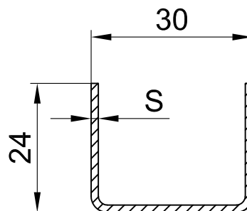
арм. 24x30x24
