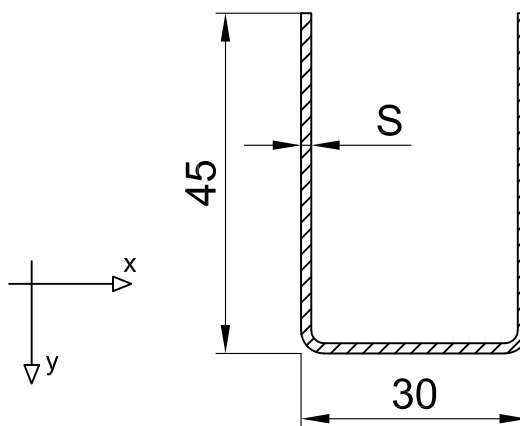
арм. 45x30x45
