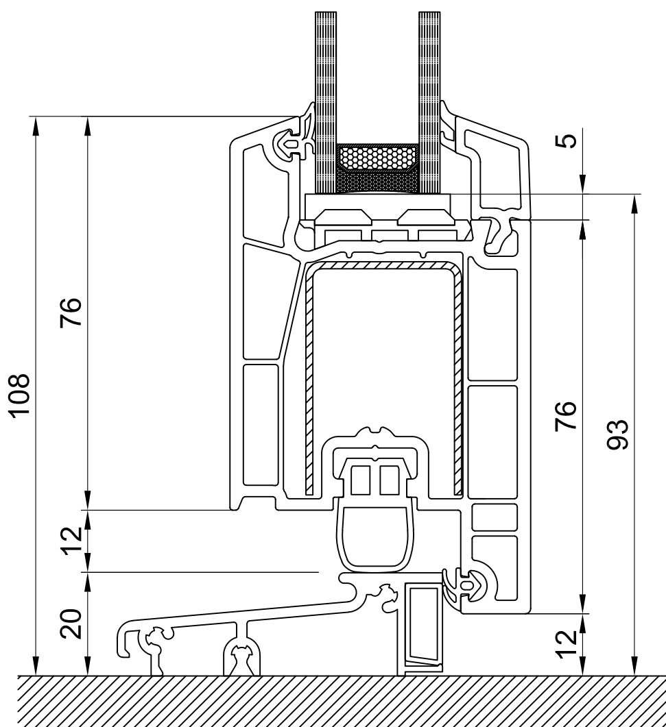
СХЕМА УЗЛА 400565 СТВОРКА ДВЕРНАЯ 96мм ПОРОГ АЛЮМИНИЕВЫЙ
