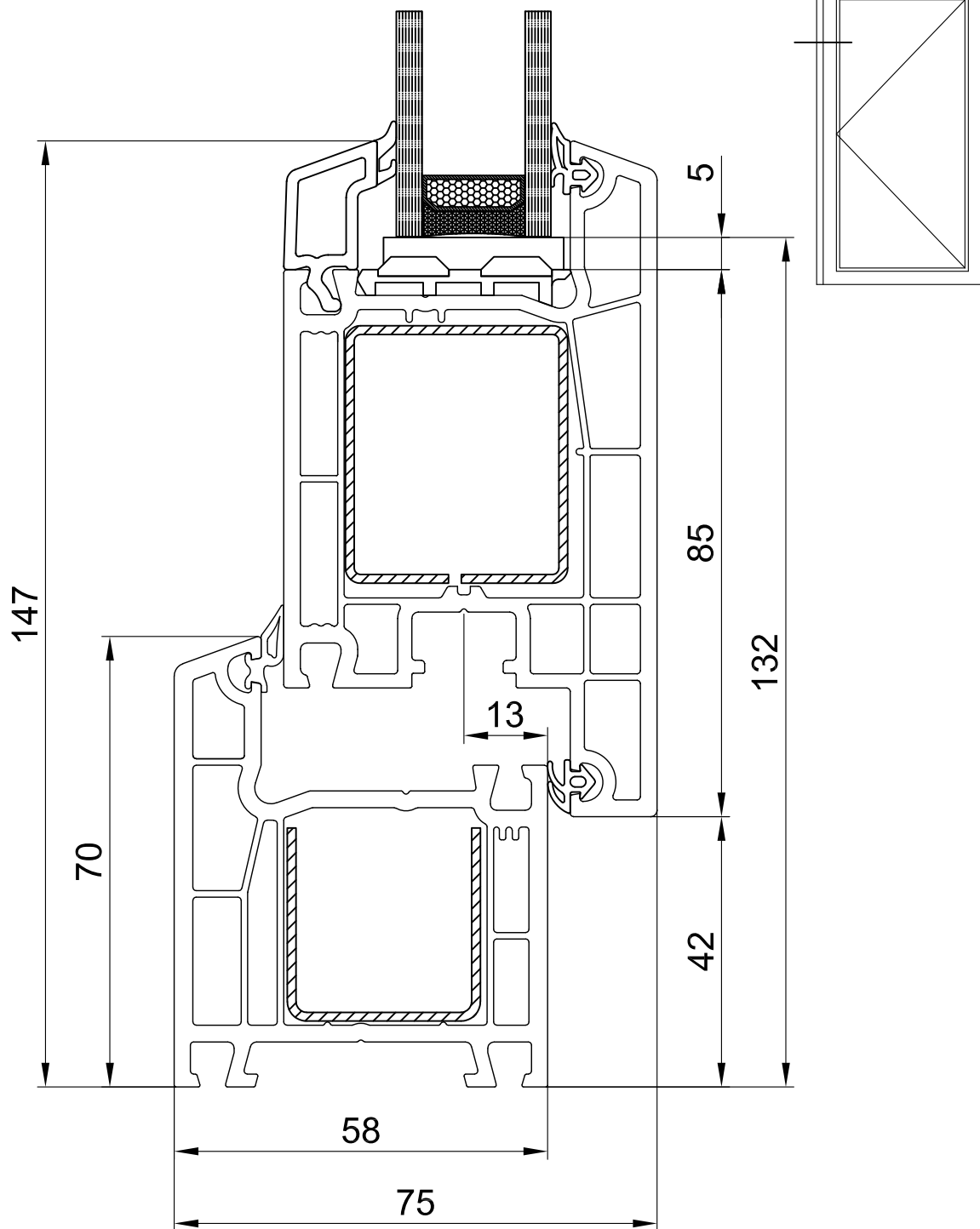
СХЕМА УЗЛА 400665 РАМА 70мм 400465 СТВОРКА ДВЕРНАЯ 105мм
