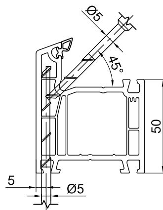
400665 рама 70мм
