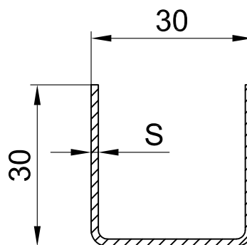
арм. 30x30x30
