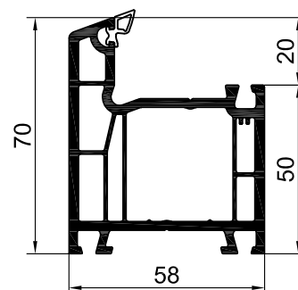
400665 рама 70мм
