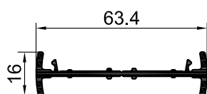
111300 соединитель Н-образный
