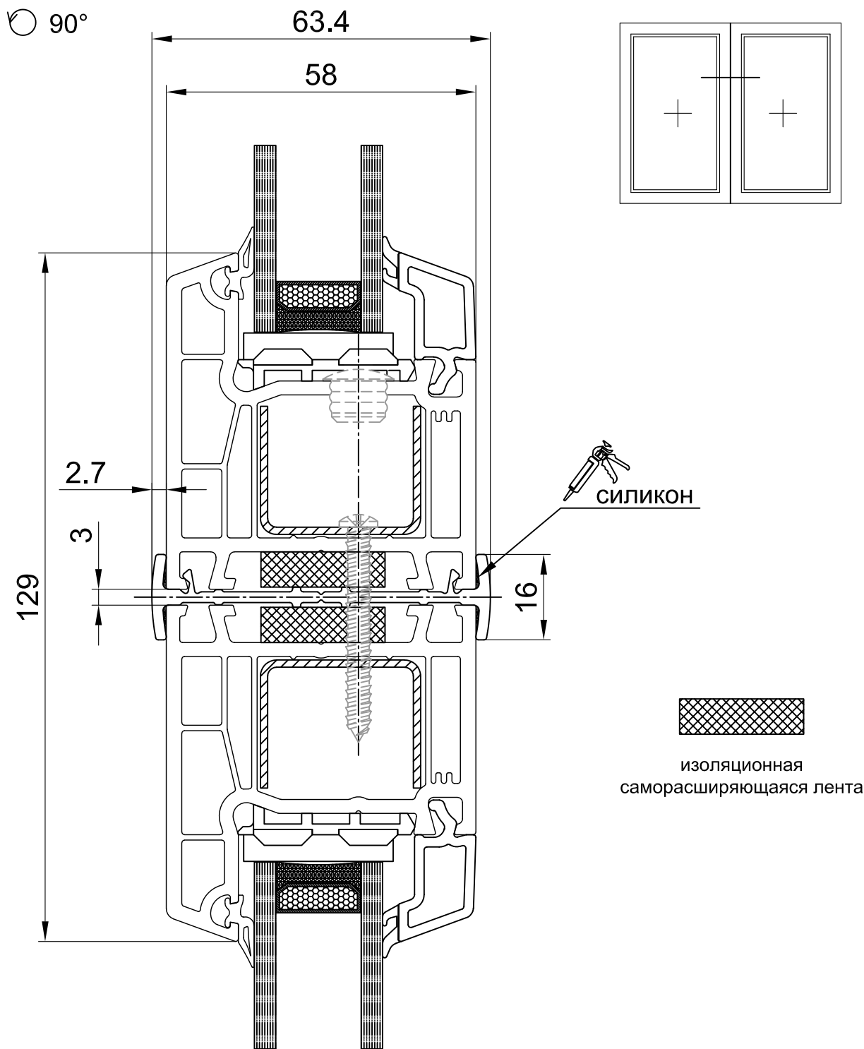
СХЕМА УЗЛА 400165 РАМА 63мм 111300 соединитель Н-образный 400165 РАМА 63мм
