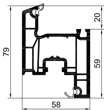
400265 створка оконная 79мм
