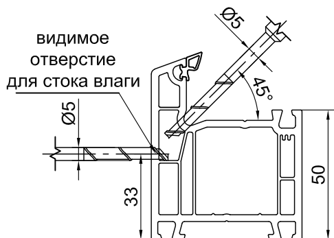
400665 рама 70мм
