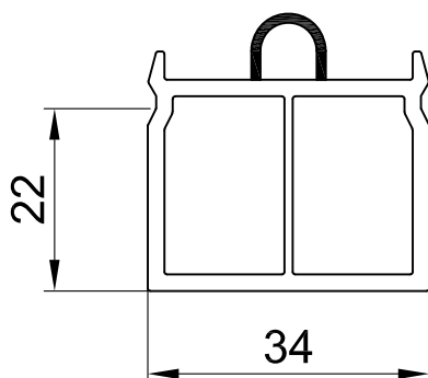
111165 VL профиль подставочный
