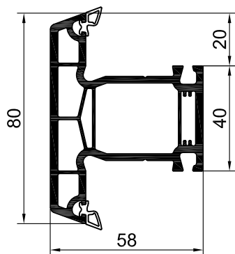
200365 импост 80мм
