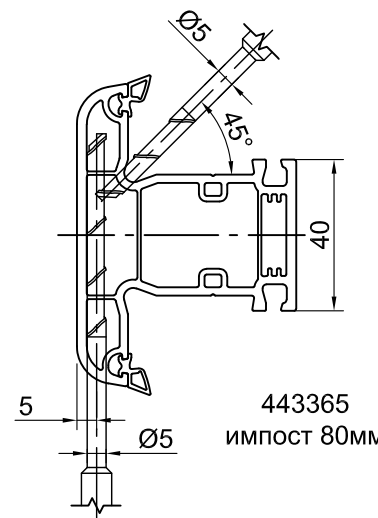
403365 импост 80мм
