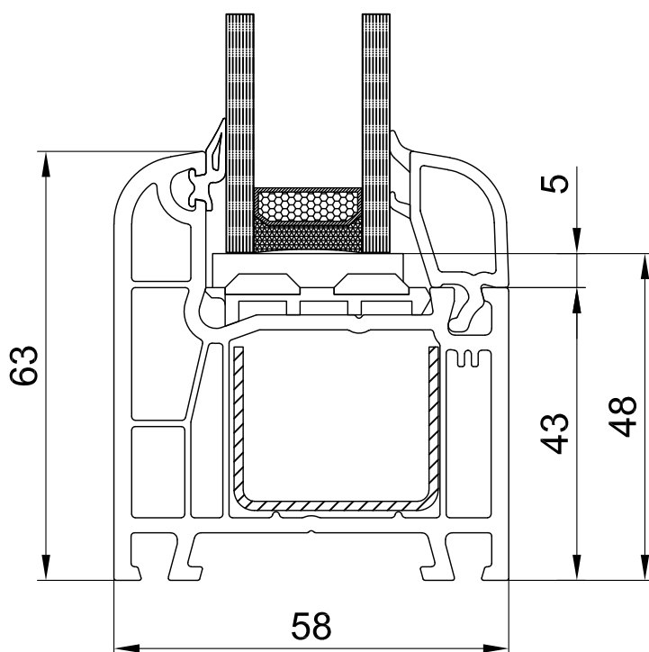
441165 РАМА 63мм
