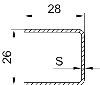
арм. 28x26x28
