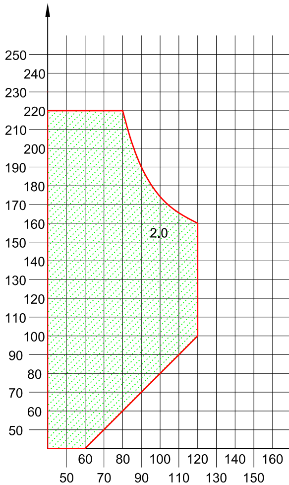
арм. 45x30x45x2.0
