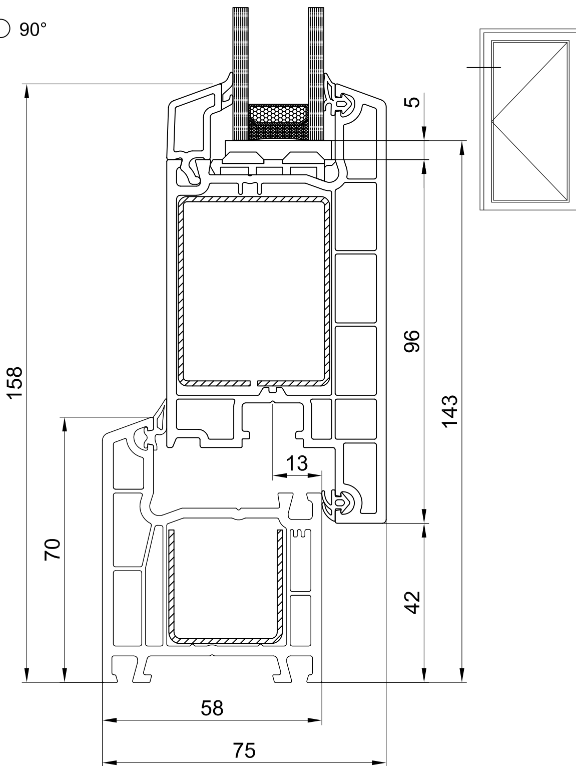
СХЕМА УЗЛА 400665 РАМА 70мм 401465 СТВОРКА ДВЕРНАЯ 116мм
