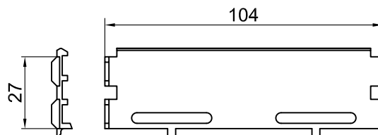
200865 штапик под заполнение 24мм
