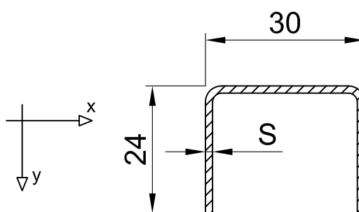
арм. 24x30x24
