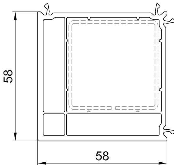
111665 соединитель 90°
