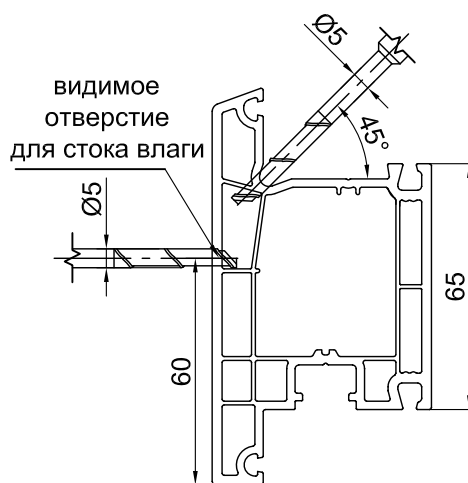
400465 створка дверная 105мм
