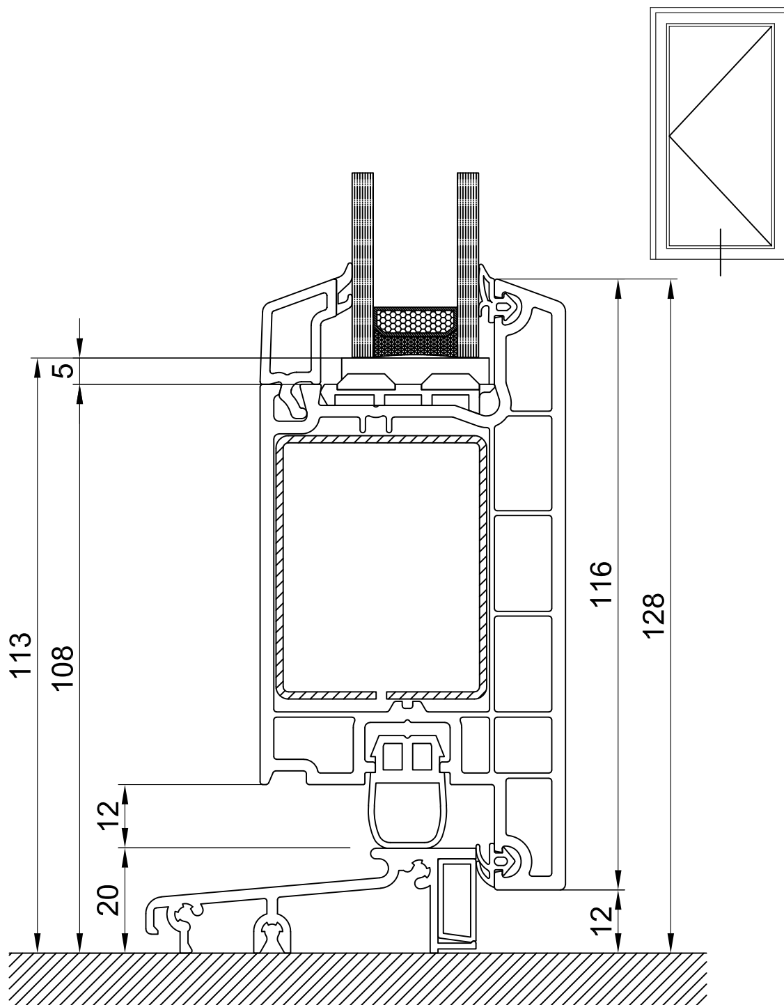
СХЕМА УЗЛА 401465 СТВОРКА ДВЕРНАЯ 116мм ПОРОГ АЛЮМИНИЕВЫЙ
