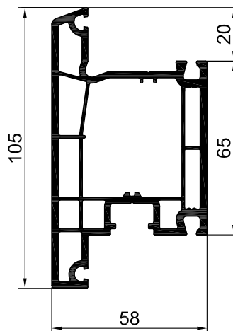
400465 створка дверная 105мм
