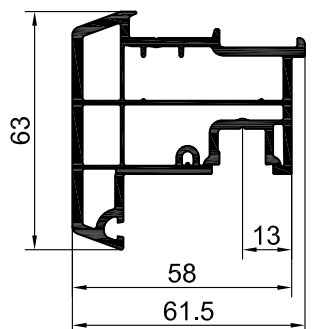
111265(13) фальшимпост (штульп)
