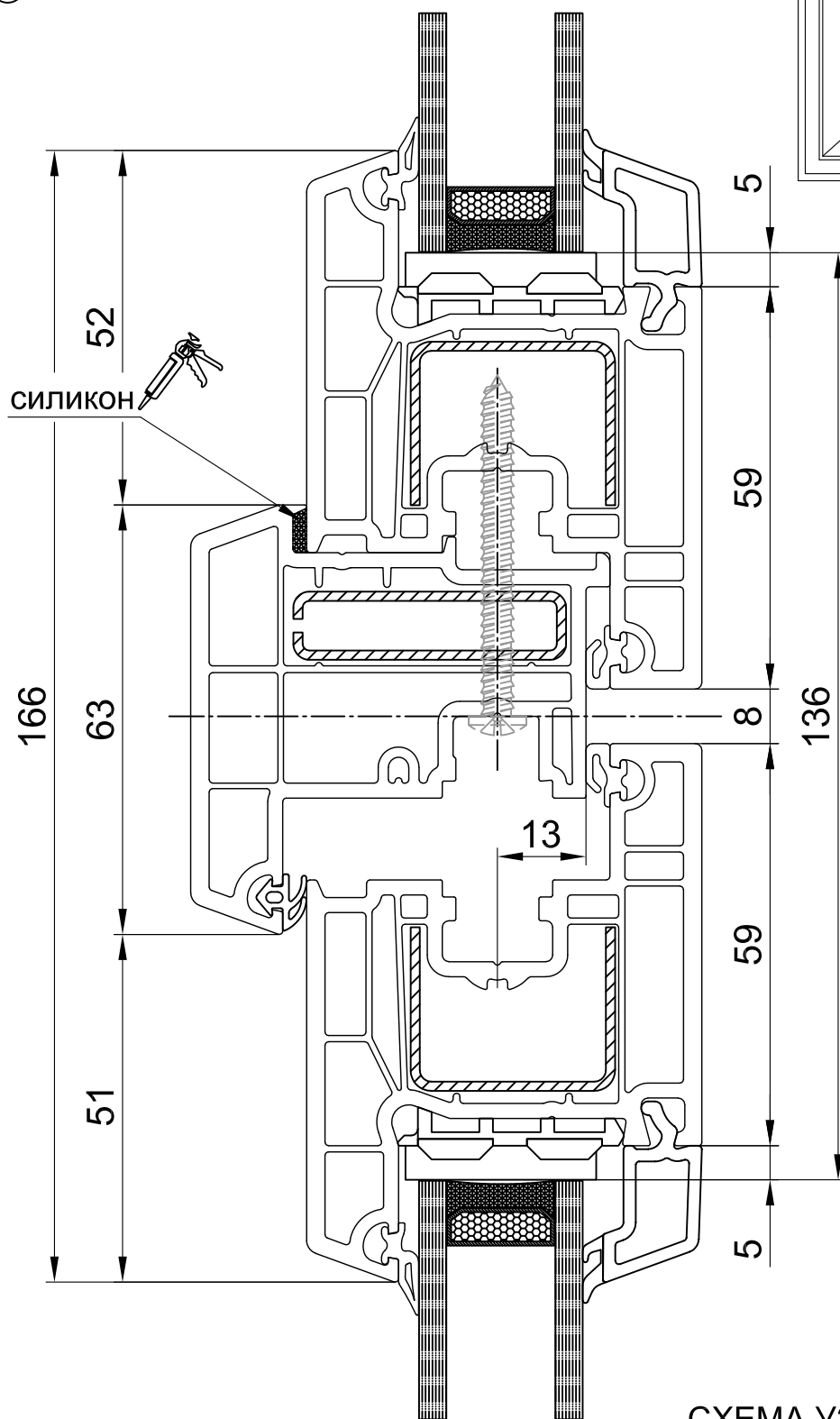
СХЕМА УЗЛА 111265(13) ШТУЛЬП 400265 СТВОРКА 79мм
