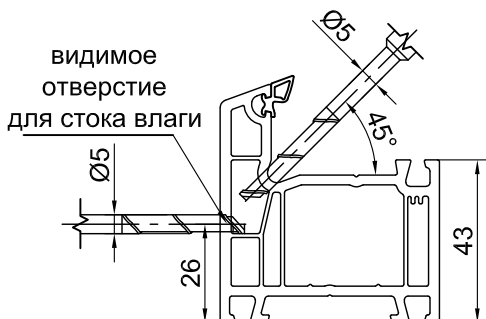
400165 рама 63мм
