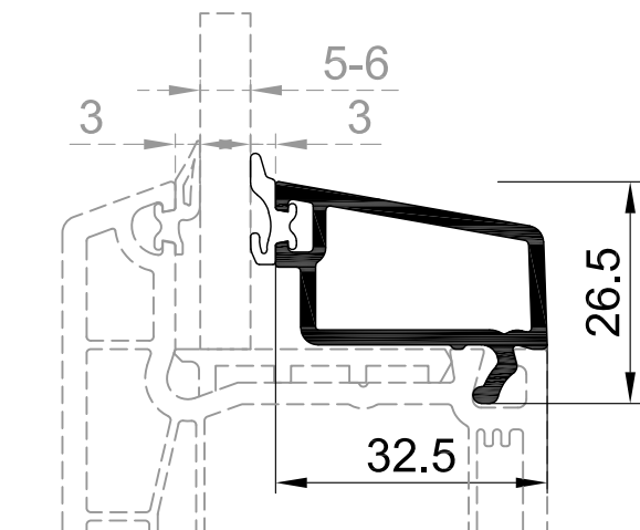
201065 штапик под заполнение 5-6мм
