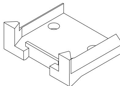
14-33 соединитель импоста 20-33 (пластик)
