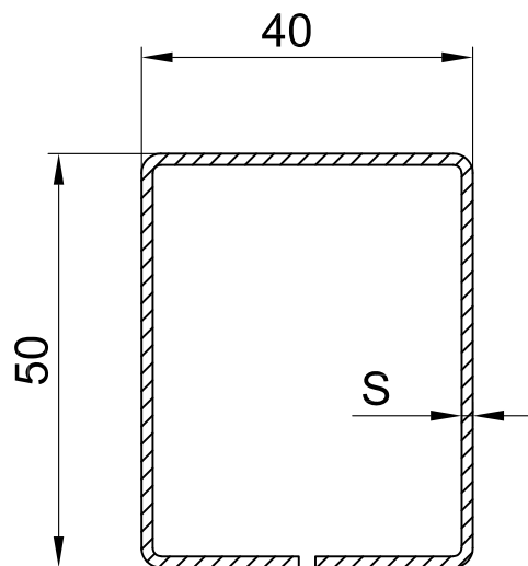
арм. 50x40x50x40
