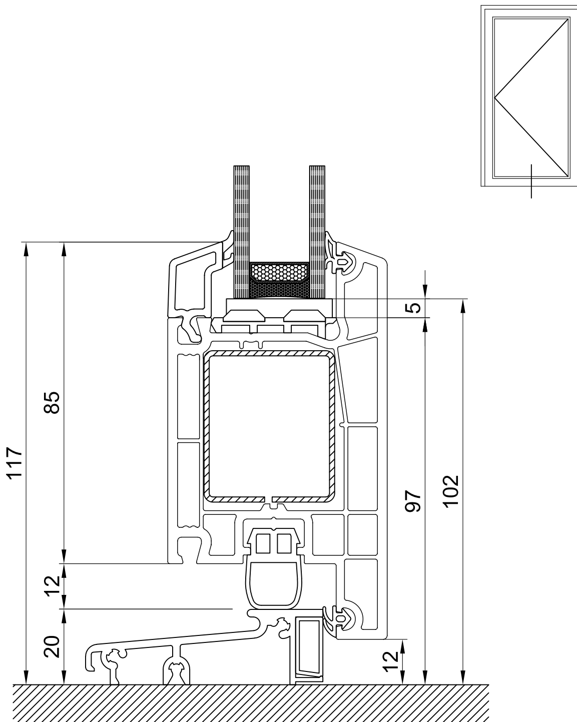
СХЕМА УЗЛА 400465 СТВОРКА ДВЕРНАЯ 105мм ПОРОГ АЛЮМИНИЕВЫЙ
