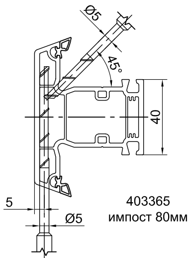
200365 импост 80мм
