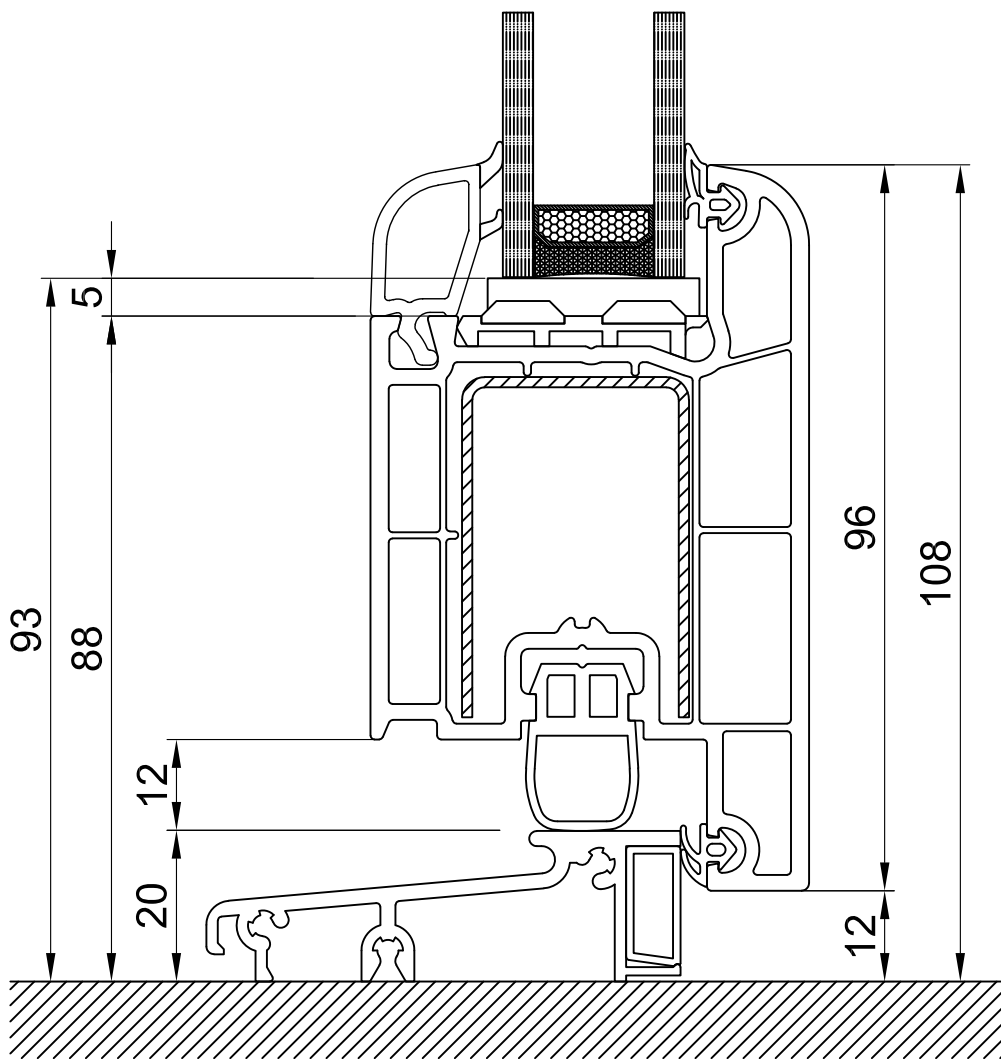
СХЕМА УЗЛА 440465 СТВОРКА ДВЕРНАЯ 96мм ПОРОГ АЛЮМИНИЕВЫЙ
