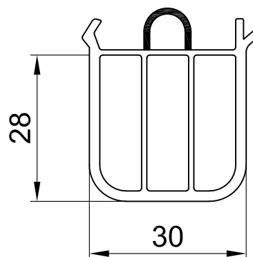
111100 профиль транспортный
