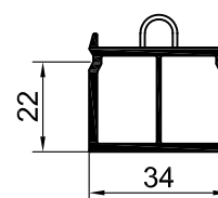
111165 VL профиль подставочный
