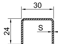
арм. 24x30x24
