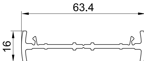
111300 соединитель H-образный
