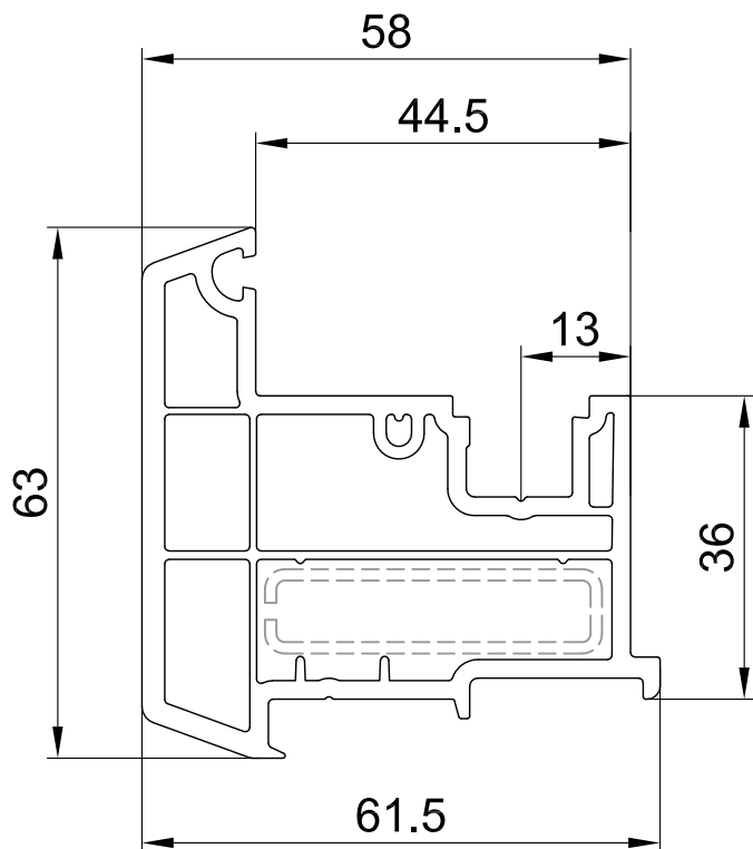
111265(13) шульп
