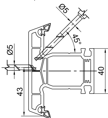
200365 импост 80мм
