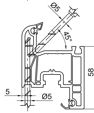
441265 створка оконная 78мм
