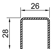
арм. 28x26x28
