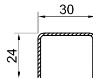
арм. 24x30x24
