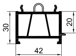
551165 VL профиль подставочный
