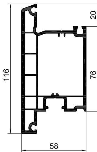
401465 створка дверная 116мм
