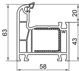
441165 РАМА 63мм
