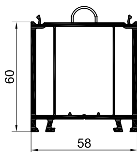
111865 расширитель 60мм
