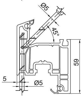
400265 створка оконная 79мм
