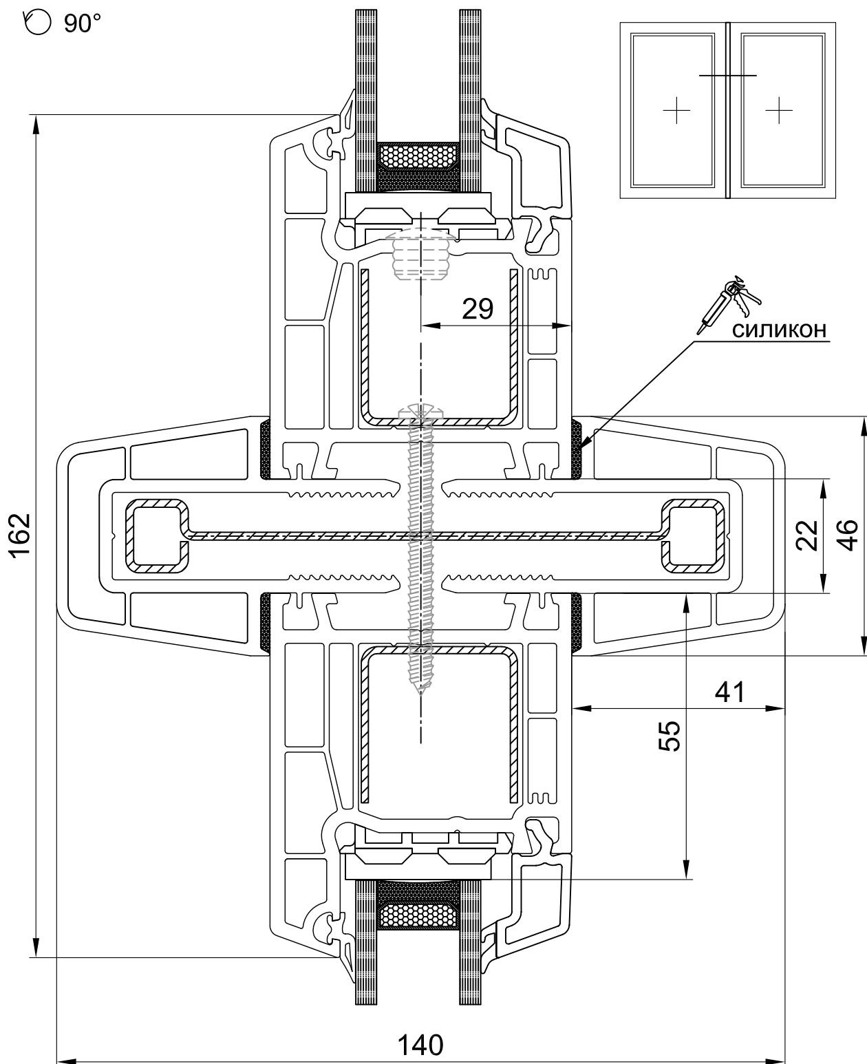
СХЕМА УЗЛА 400665 РАМА 70мм 111965 соединитель статический 400665 РАМА 70мм
