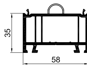
111765 расширитель 35мм
