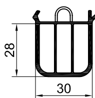
111100 профиль транспортировочный
