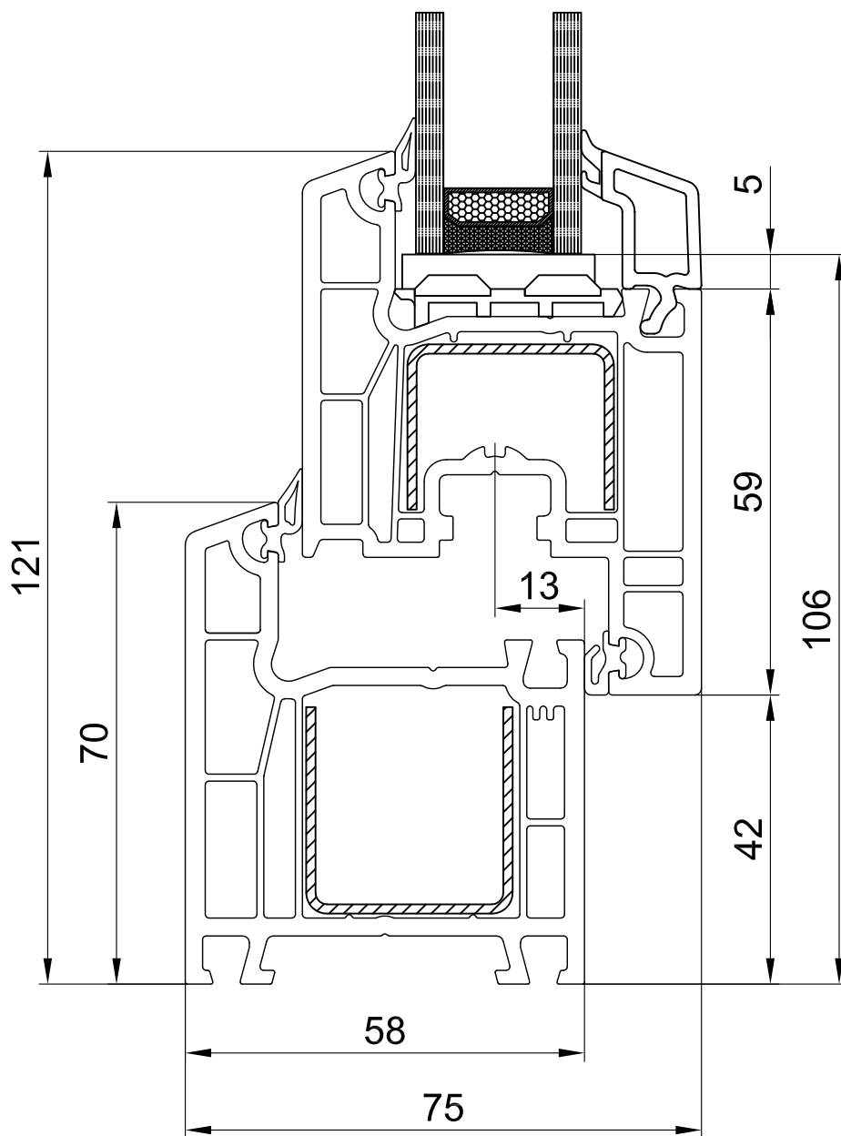
СХЕМА УЗЛА 400665 РАМА 70мм 400265 СТВОРКА 79мм
