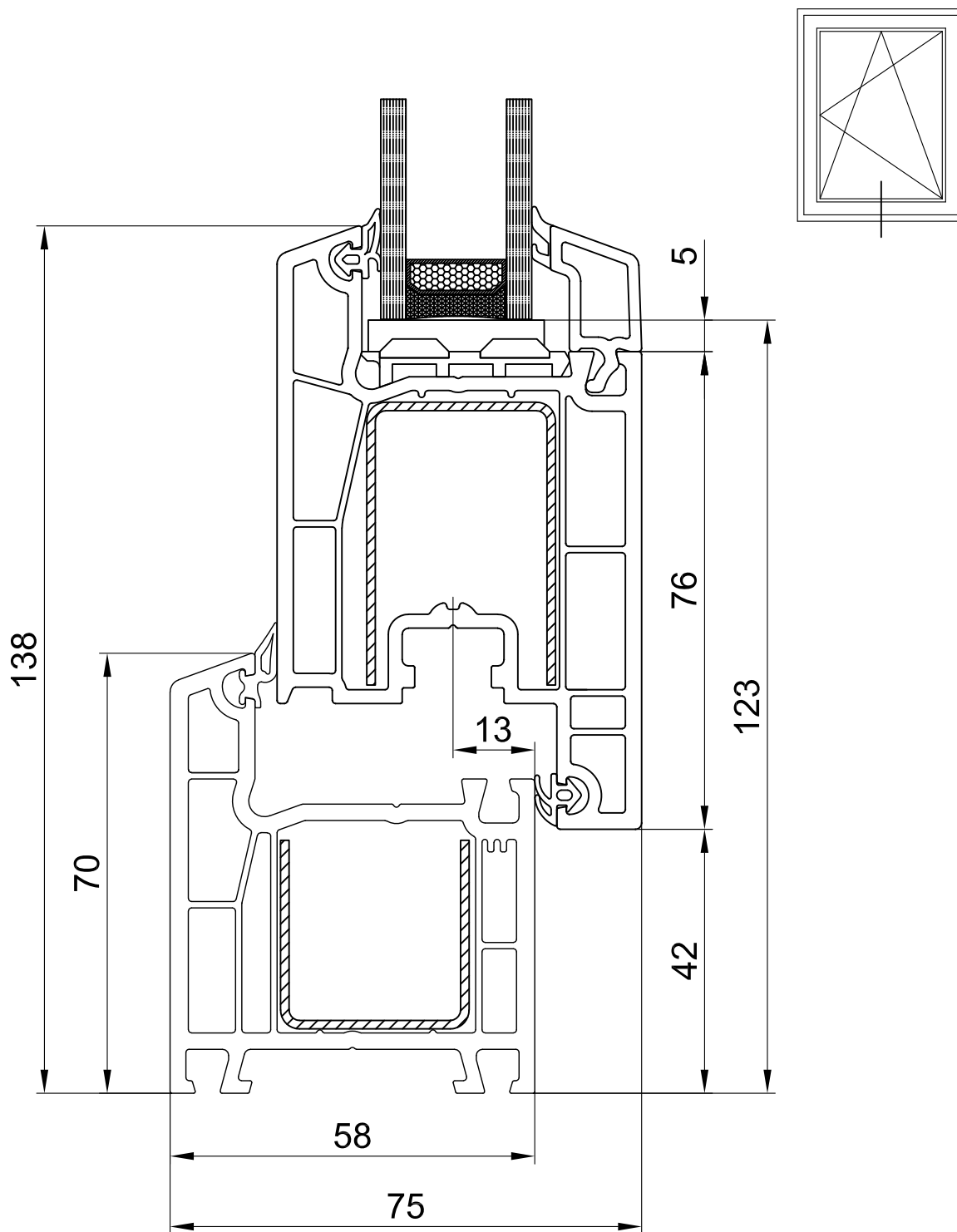
СХЕМА УЗЛА 400665 РАМА 70мм 400565 СТВОРКА ДВЕРНАЯ 96мм
