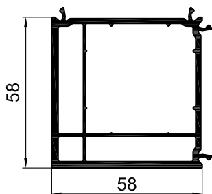
111665 соединитель 90°
